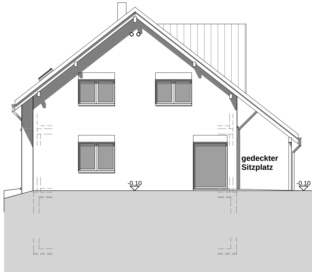
Westfassade
