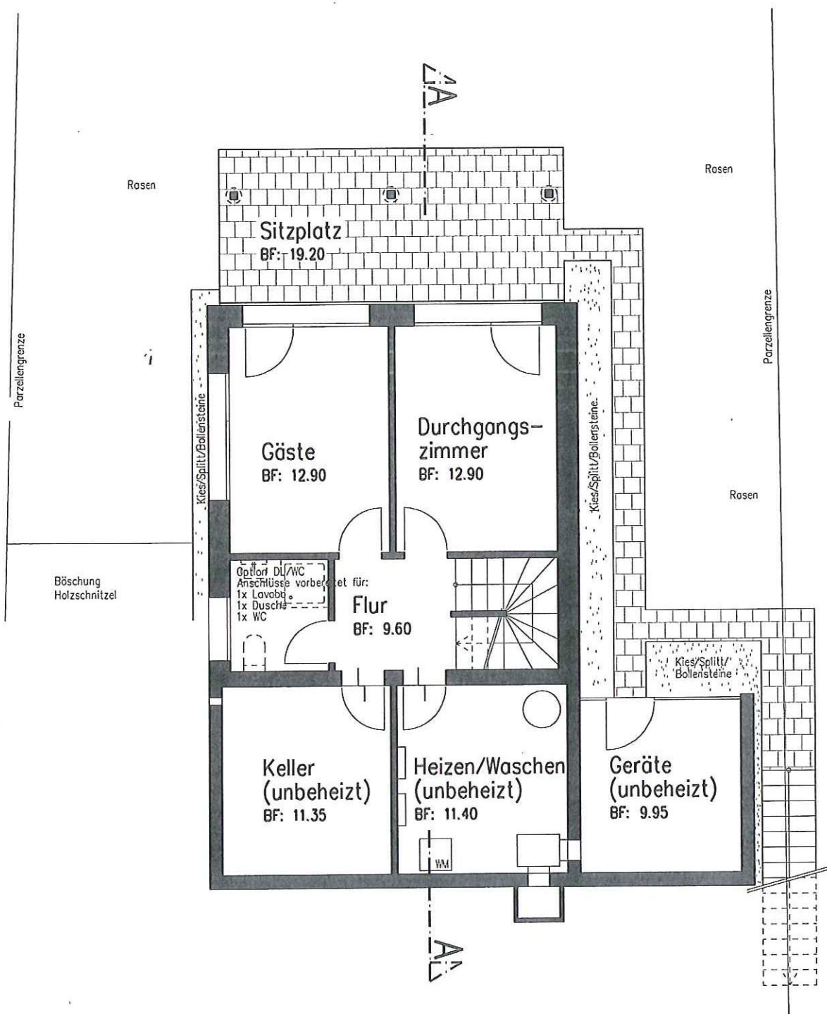
Grundriss Untergeschoss
