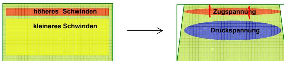
Bild 2: Die warme Zone hat ein höheres Trockenschwinden. Die Zugspannungen können Risse verursachen.
