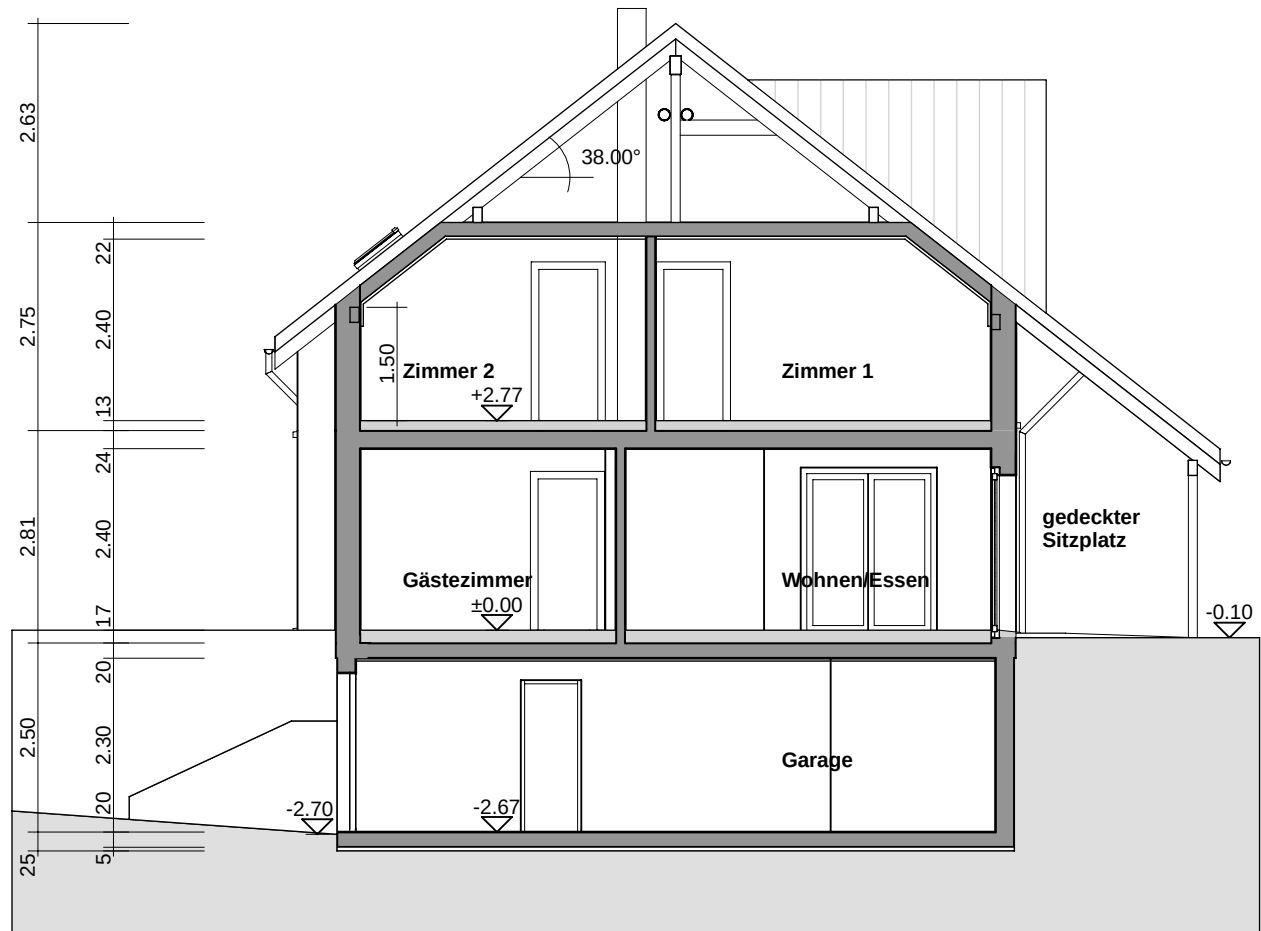
Schnitt A-A
