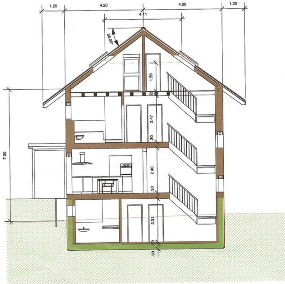
SCHNITT
