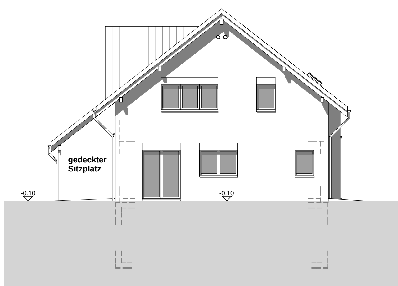
Ostfassade
