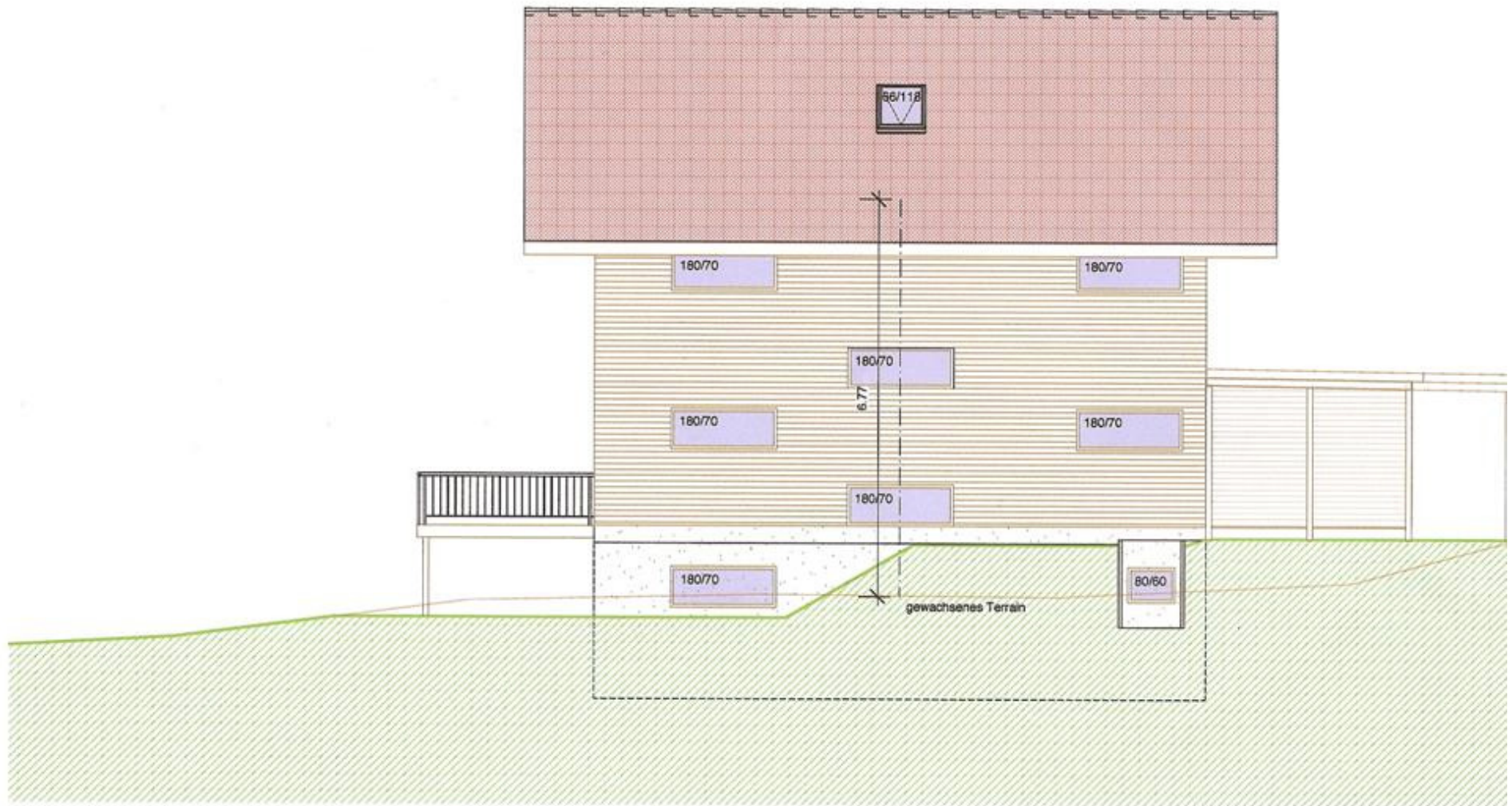
OSTFASSADE
