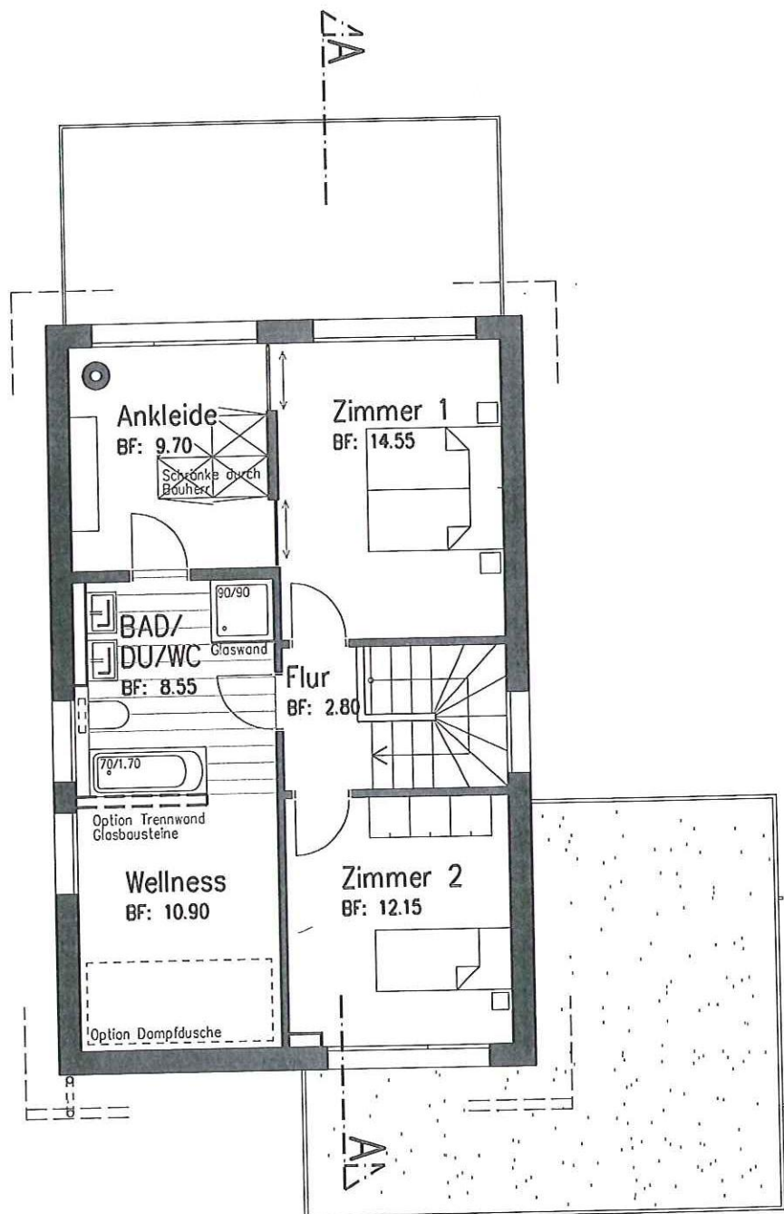
Grundriss Obergeschoss
