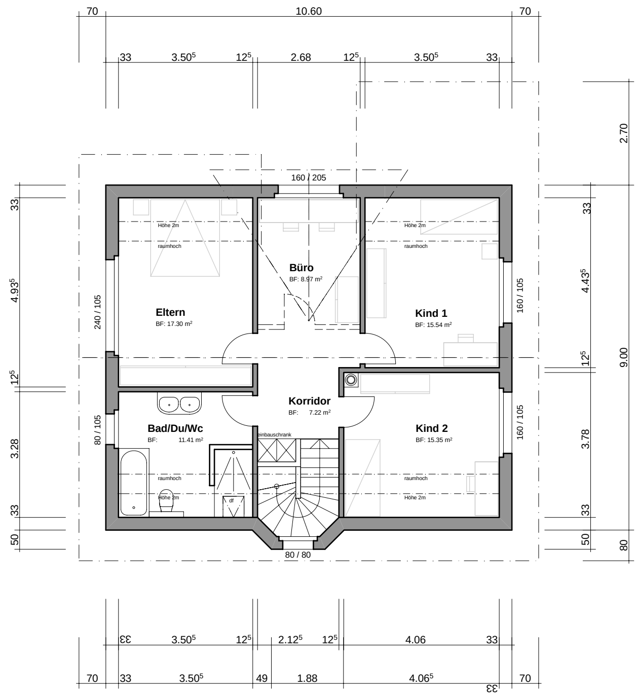
Obergeschoss
