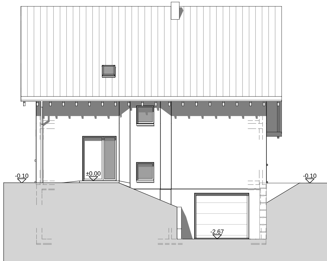
Nordfassade
