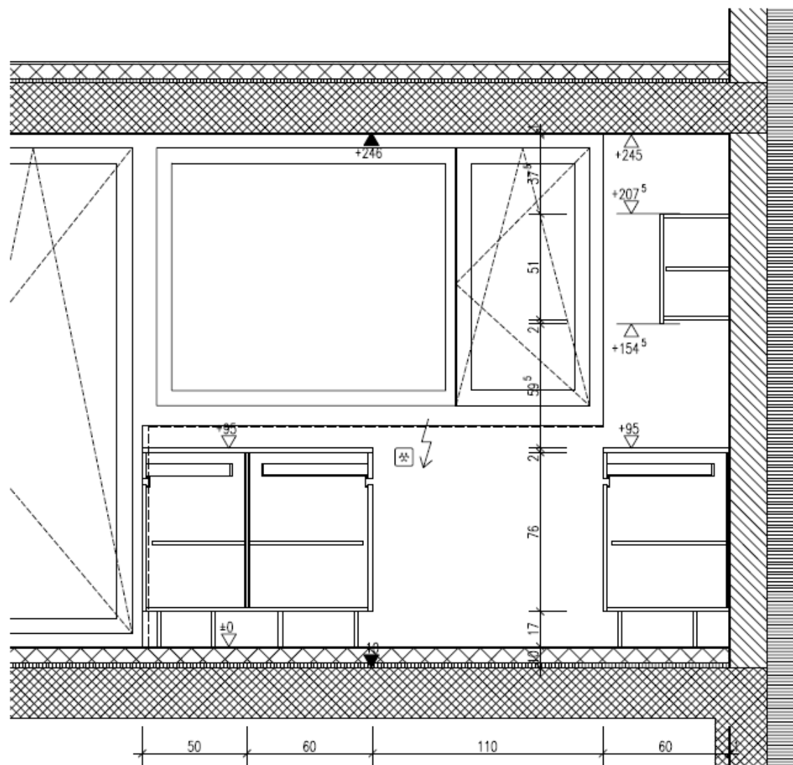
ANSICHT B
