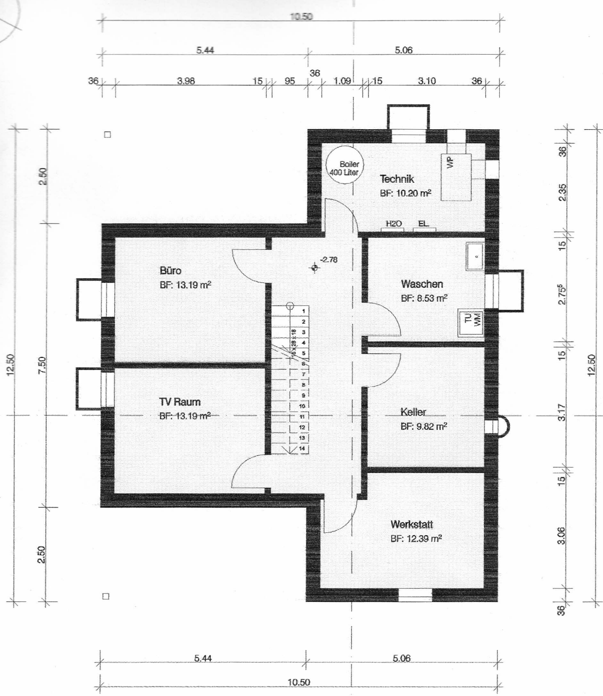
Untergeschoss
