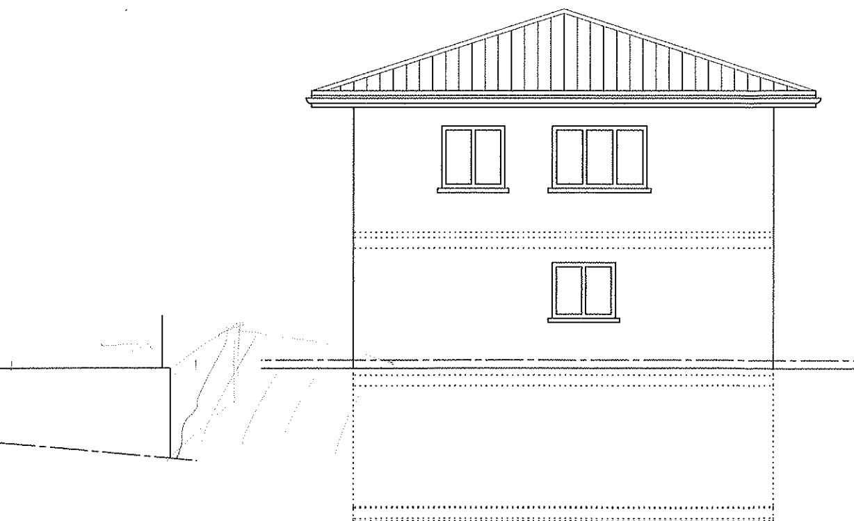
ANSICHT WEST
