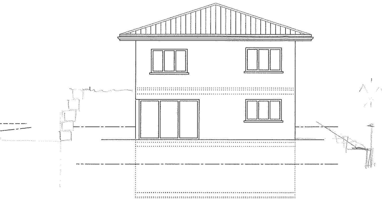
ANSICHT OST
