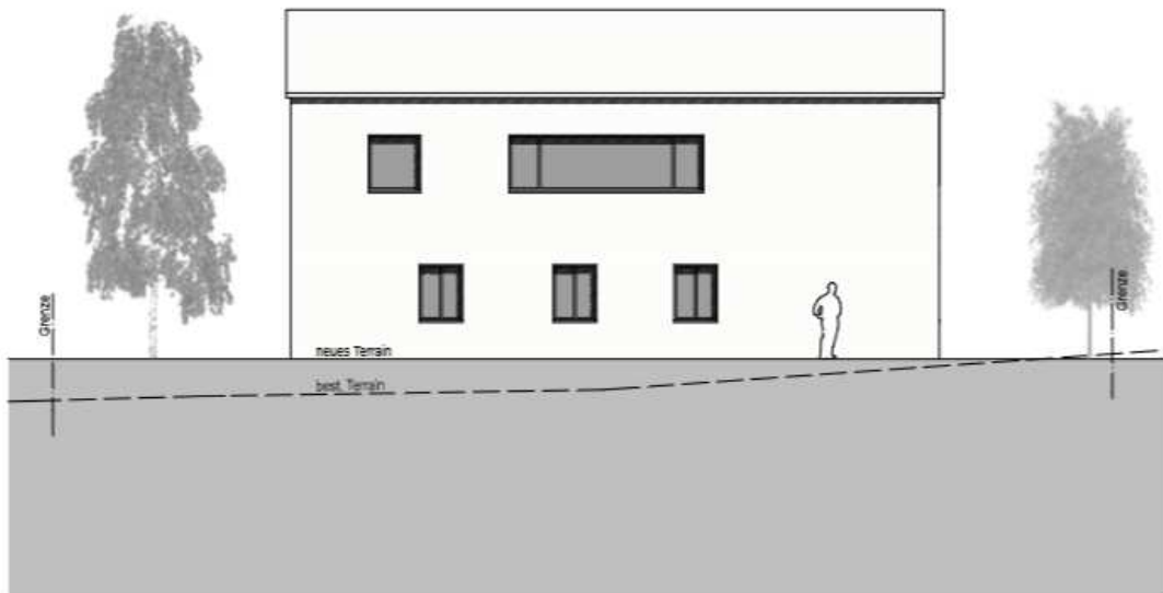
Nord-Ost Fassade
