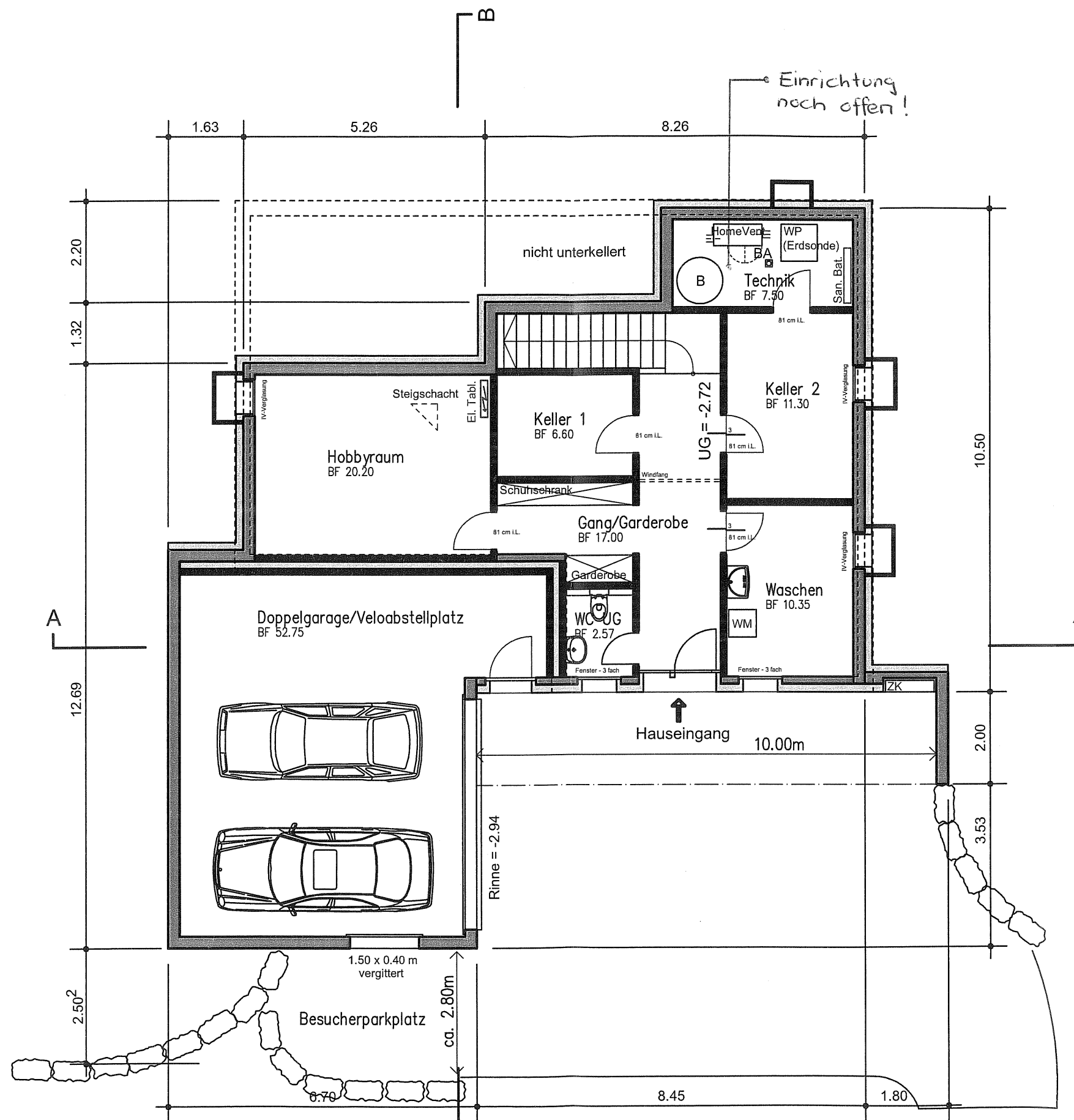
Kellergeschoss 1:100 Neubau Einfamilienhaus, Mittlere Haldenstrasse, 8196 Wil ZH
