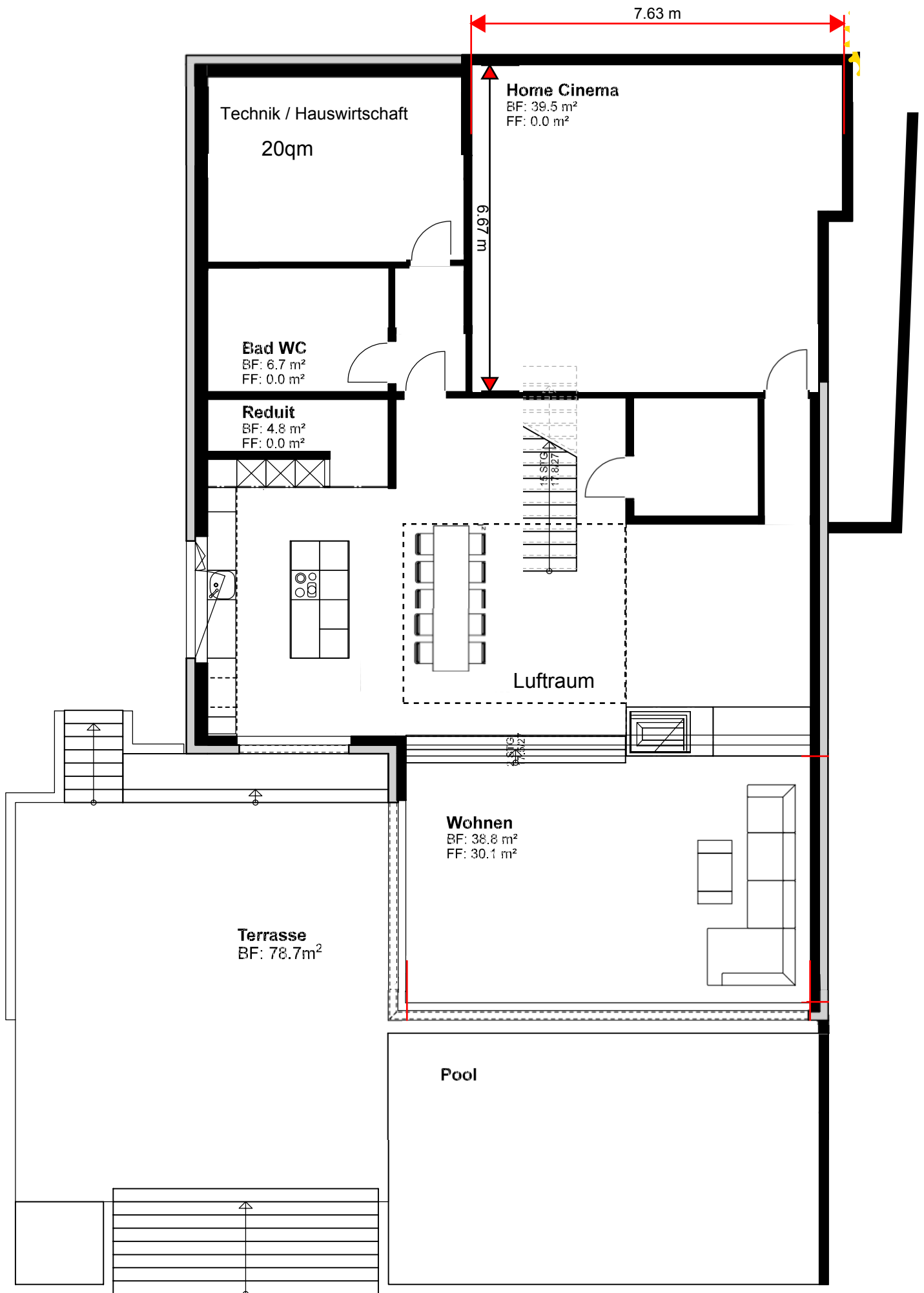
Grundriss Erdgeschoss 1:100
