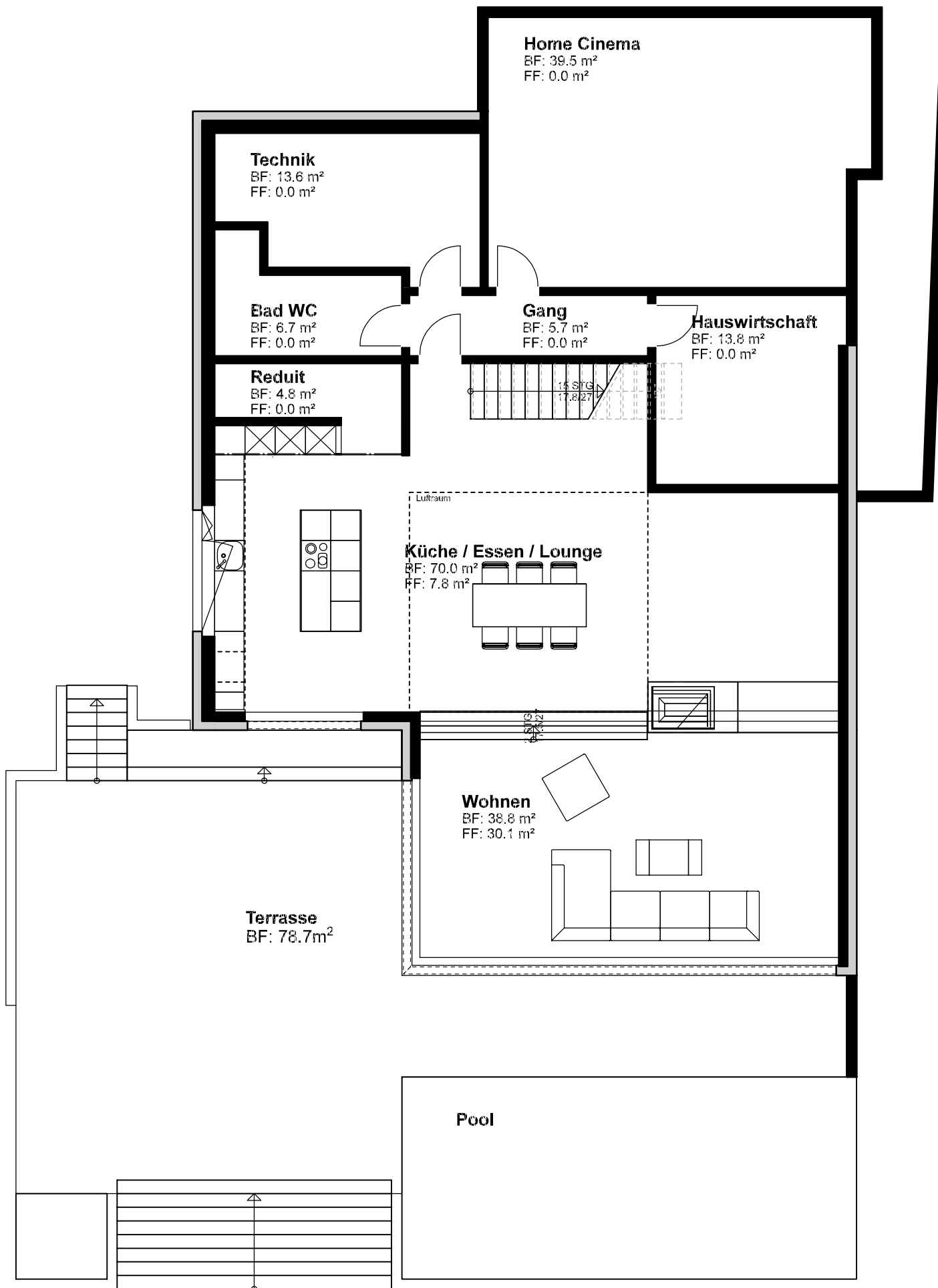
Grundriss Erdgeschoss 1:100
