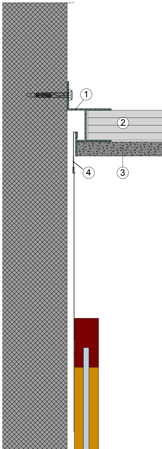
Querschnitt Decke mit Galeria - Profil, Msst. 1:2
