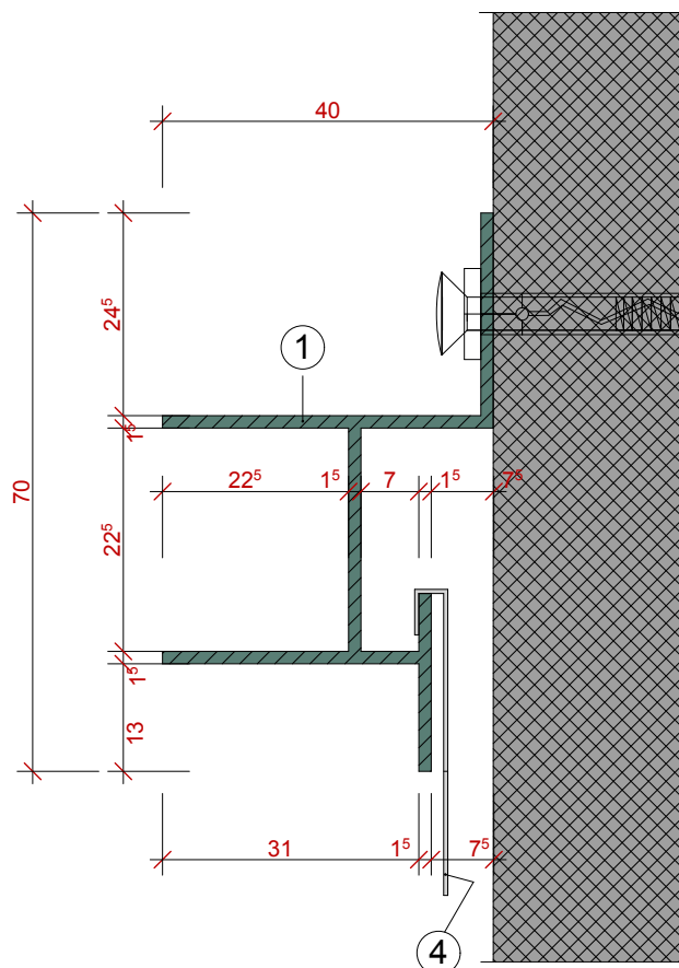
Querschnitt Galeria - Profil Msst. 1:1
