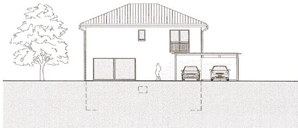
Südfassade Mst.1:200
