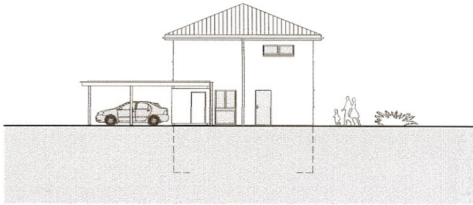
Ostfassade Mst.1:200
