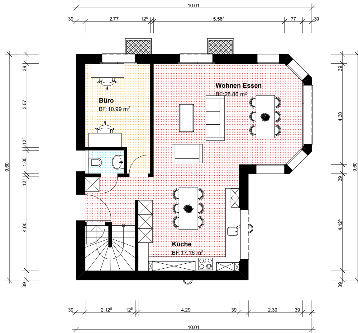
Erdgeschoss Variante 2
