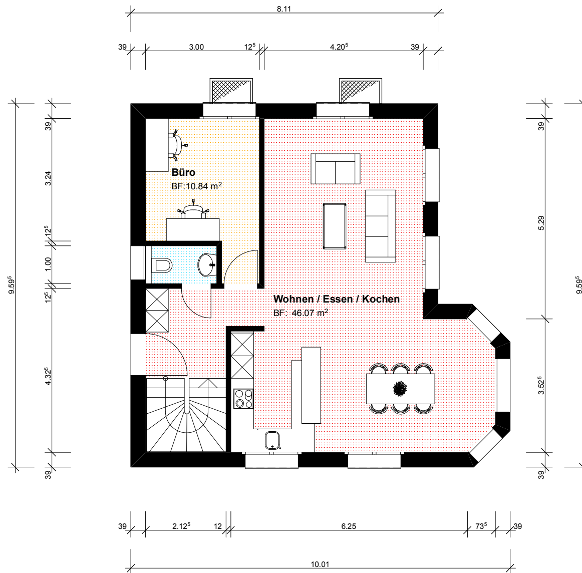
Erdgeschoss Variante 1
