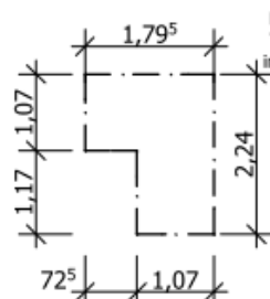
Treppenloch in der Decke über EG
