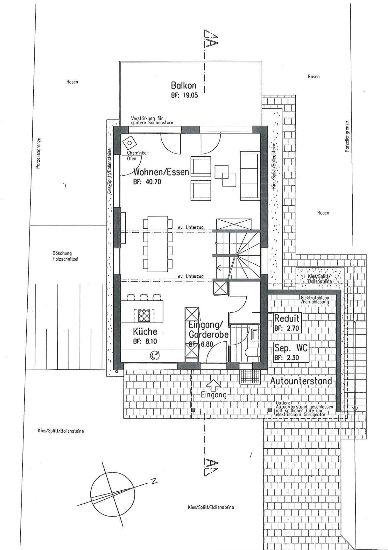
Grundriss Erdgeschoss Parz. Grösse ~459 m 2
