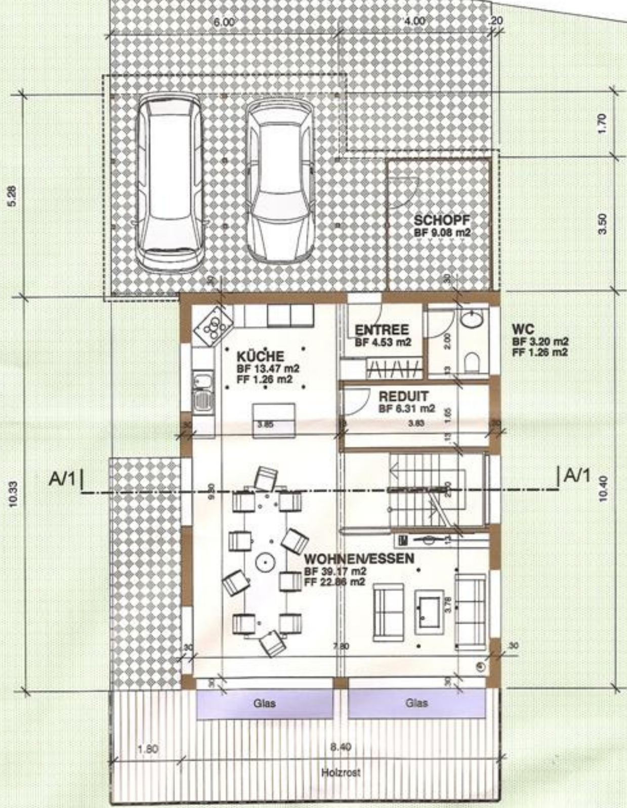
ERDGESCHOSS
