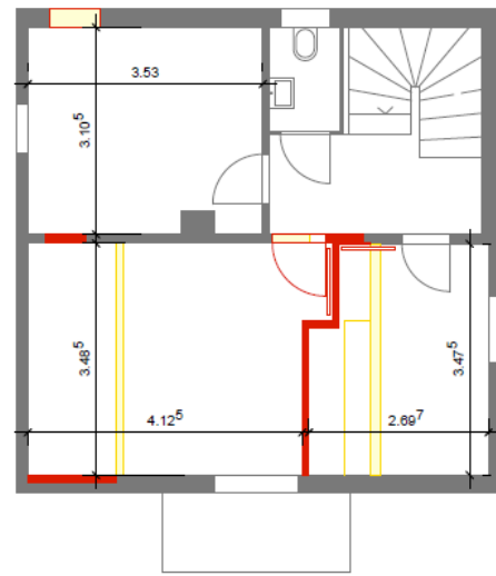
Obergeschoss
