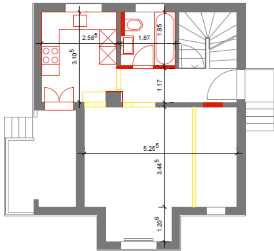
Erdgeschoss
