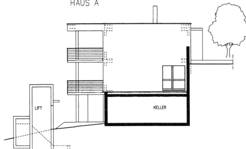
ANSICHT OST
