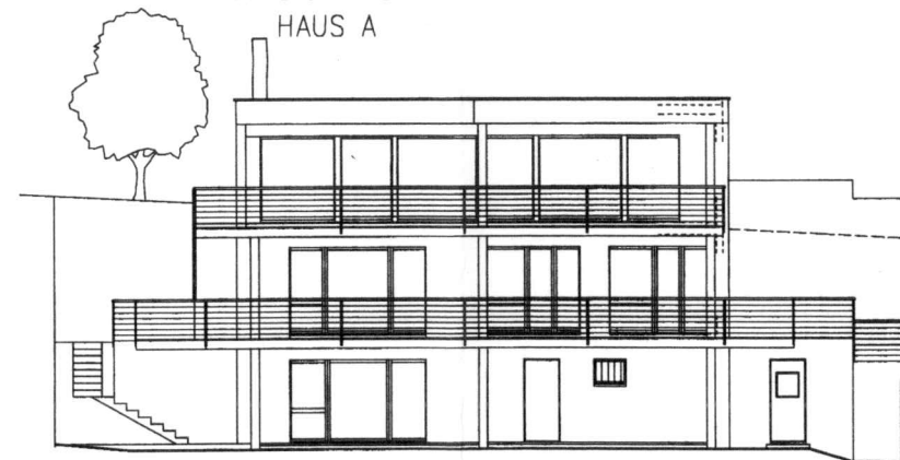
ANSICHT SÜD
