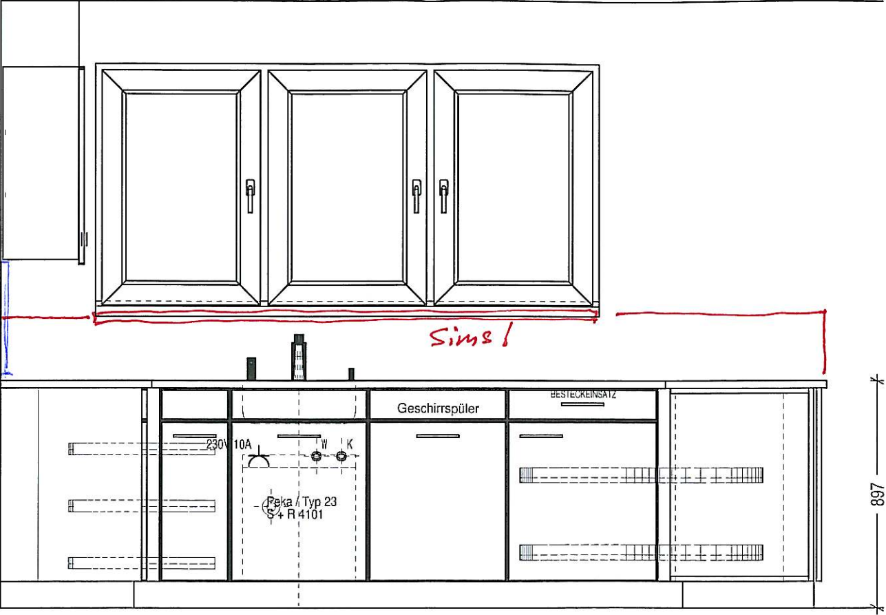
ANSICHT B
