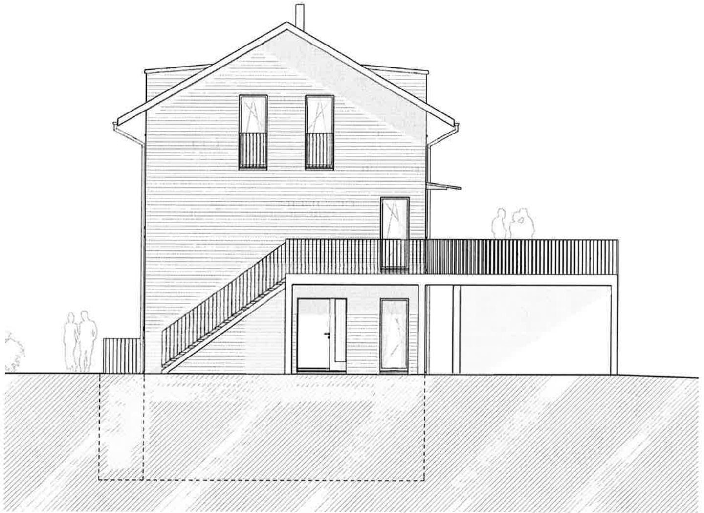
Nordwestfassade
