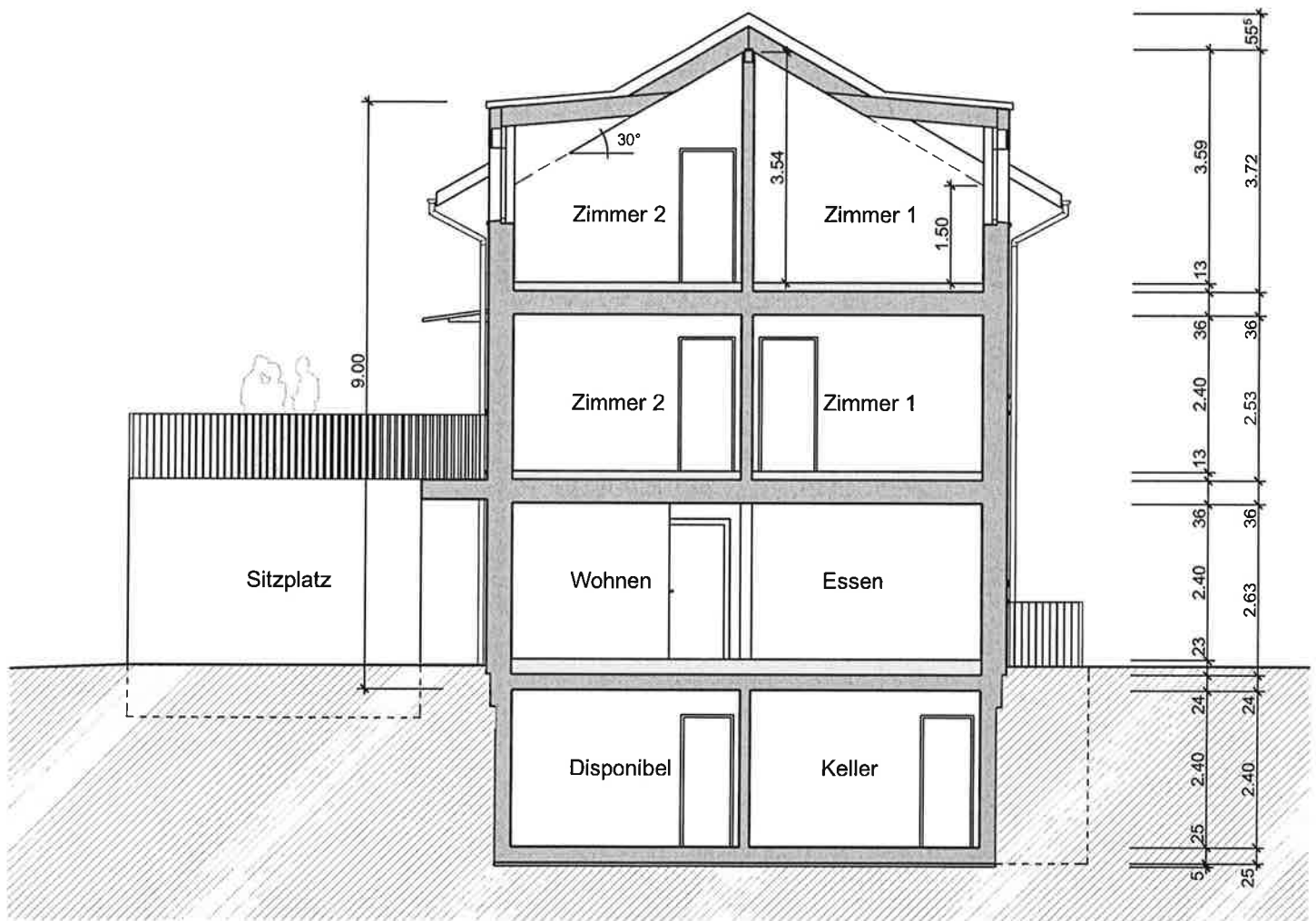
Querschnitt
