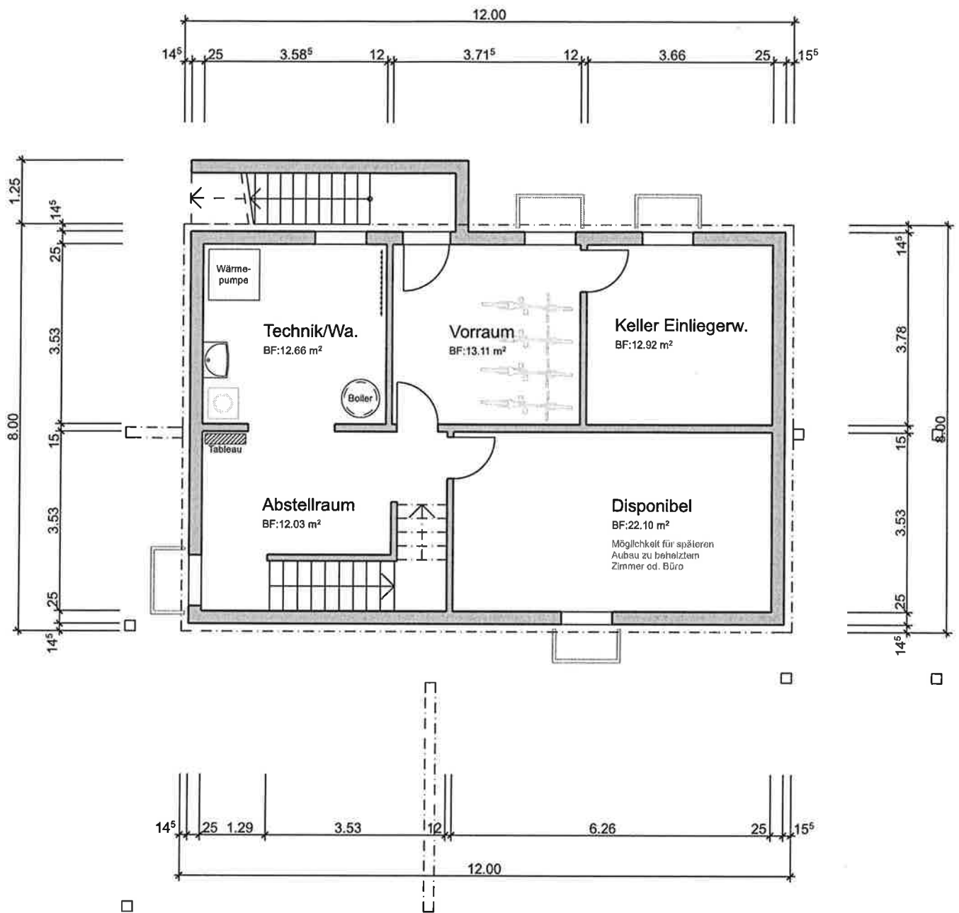
Untergeschoss
