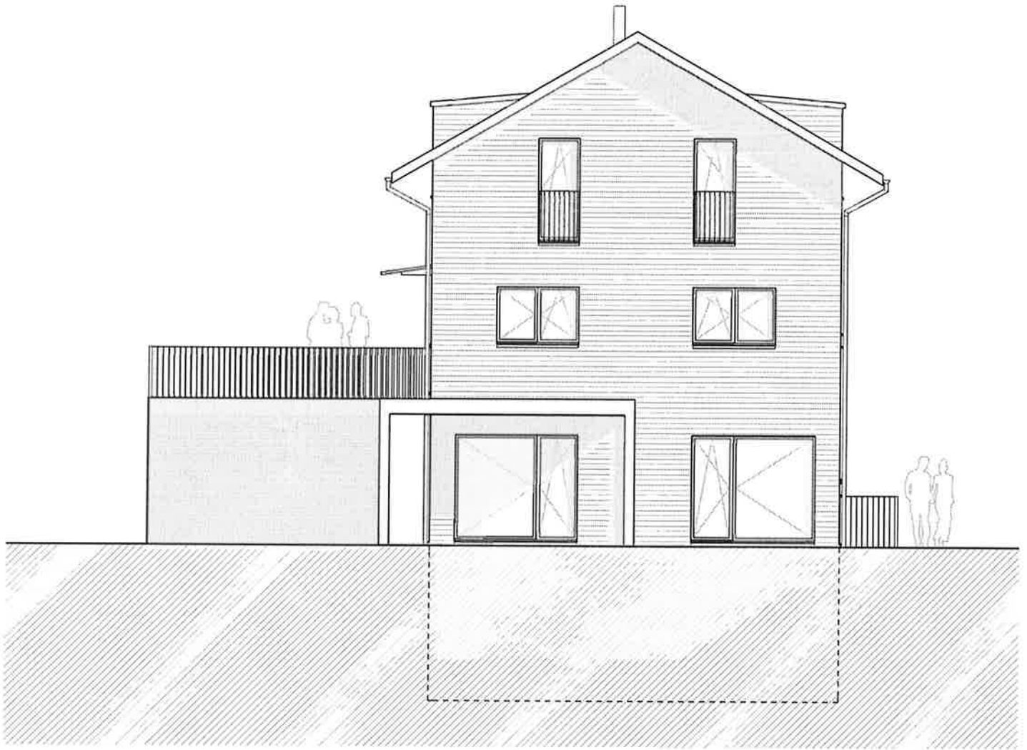
Südostfassade
