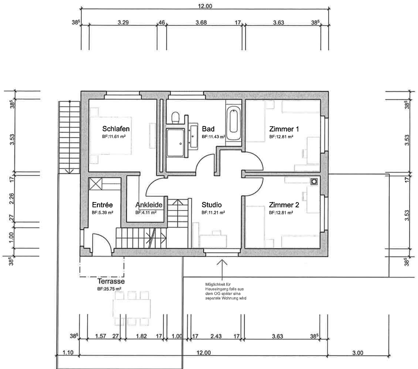
Obergeschoss
