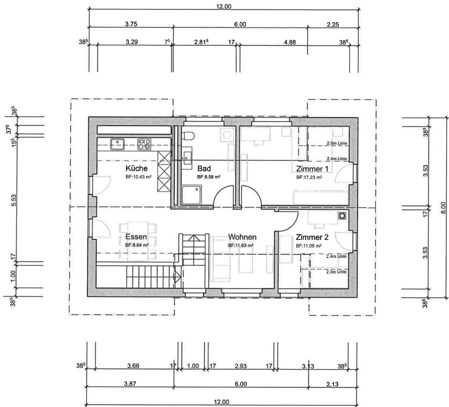
Dachgeschoss
