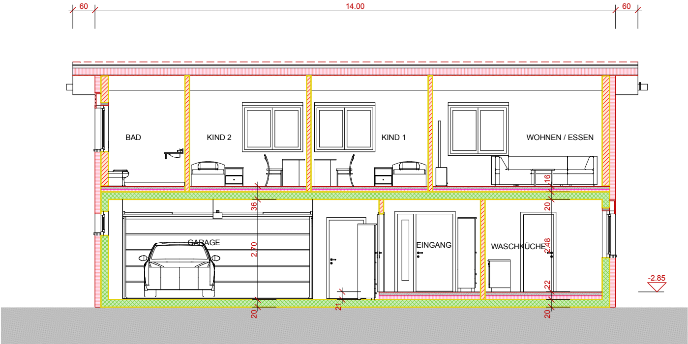
SCHNITT A-A
