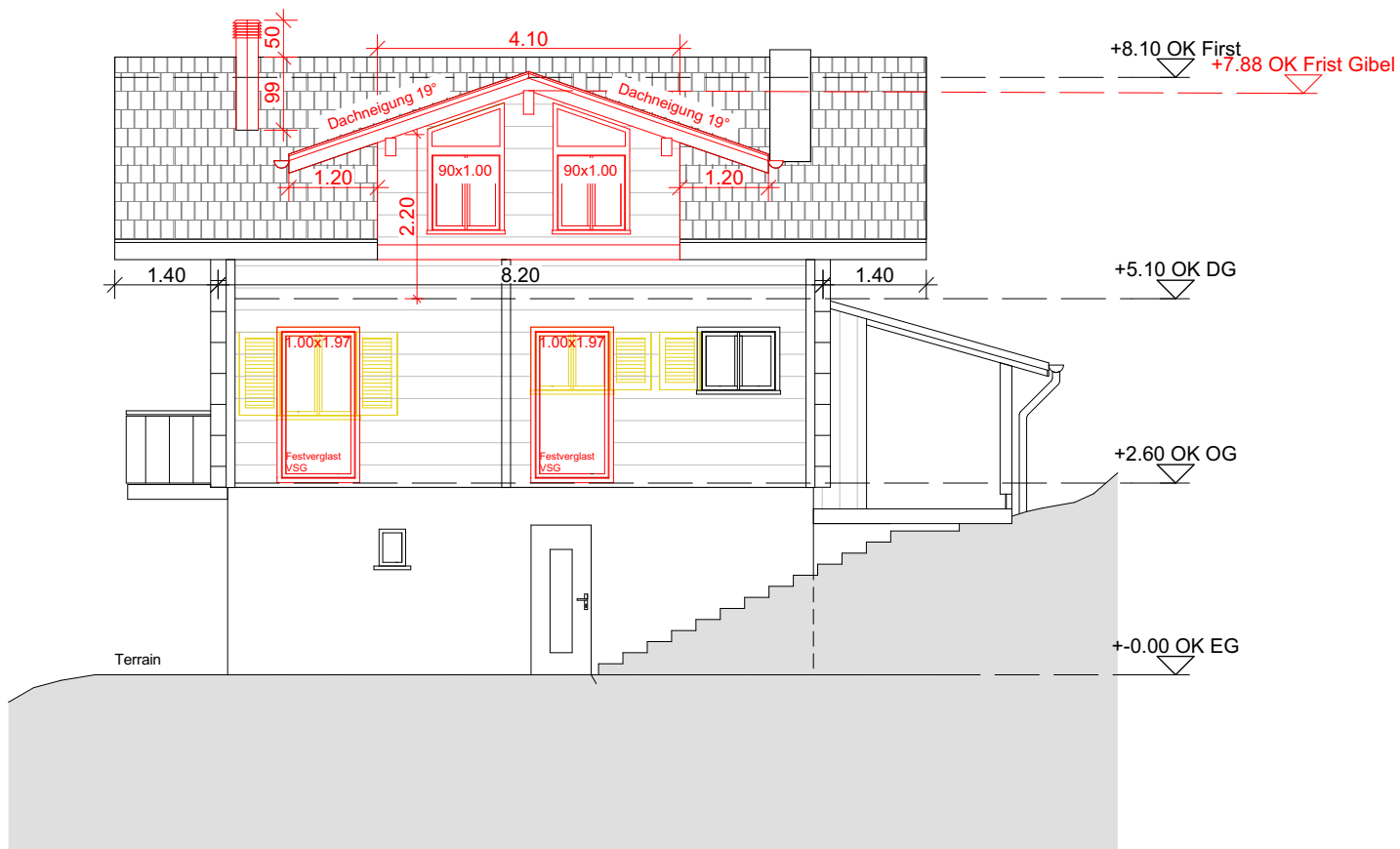
Ostfassade
