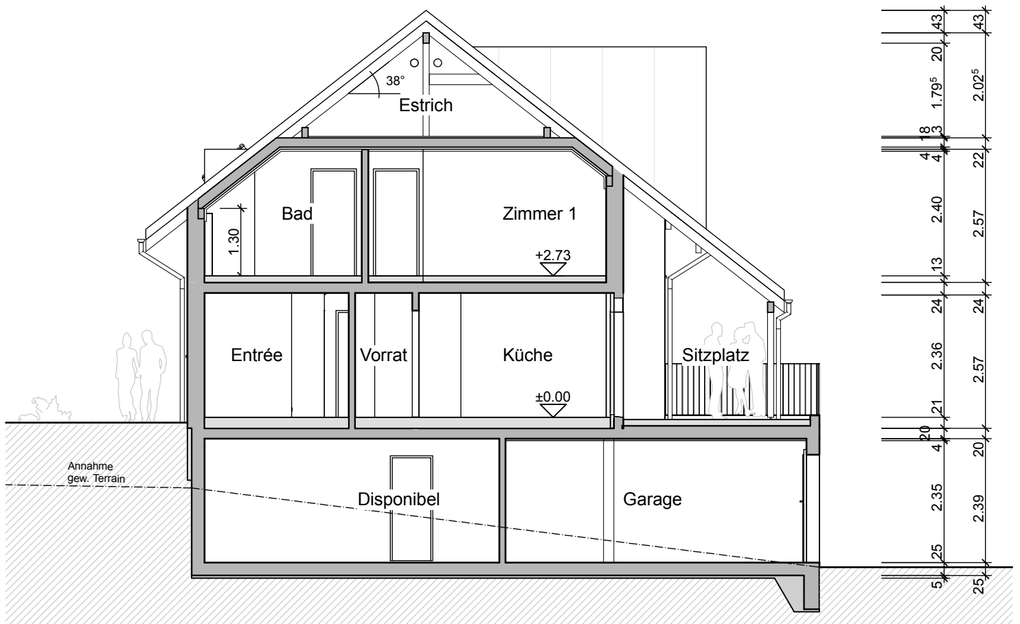
Querschnitt
