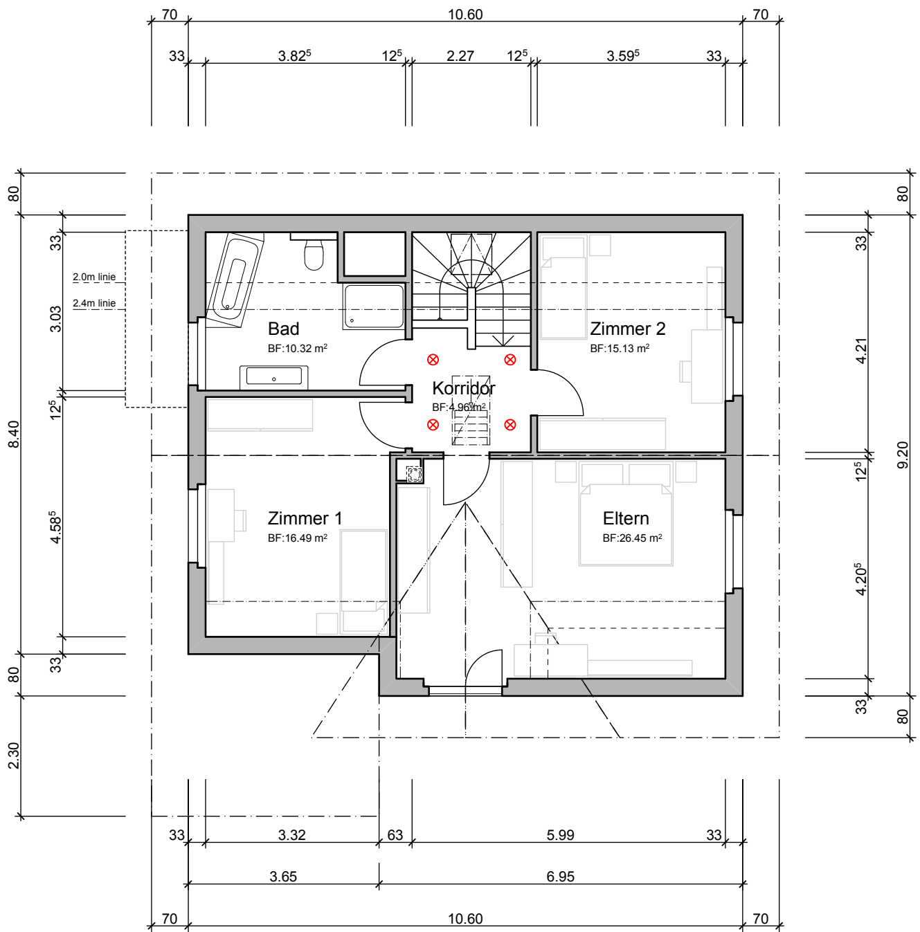
Obergeschoss
